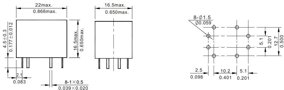
安装尺寸图 (底视图)
