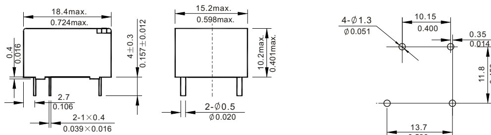
外形尺寸图
