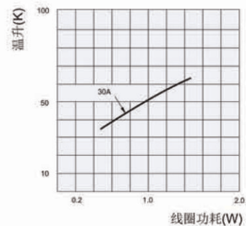
线圈温升
